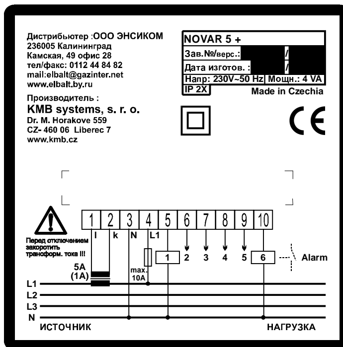
Рис.3 Регулятор НОВАР5 - разъем.
