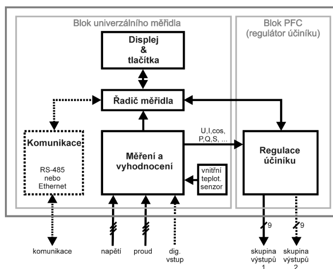
Blokové schéma regulátoru NOVAR 2400
