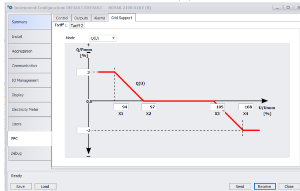
Podpora sítě v režimu Q(U) – nastavení
