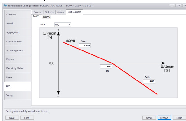
Podpora sítě v režimu U/Q – nastavení
