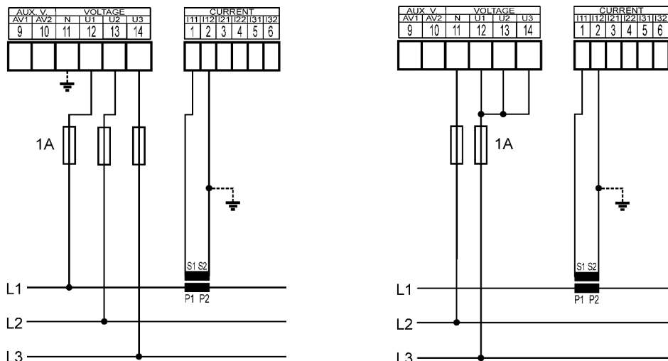
Obr. 4.23 : Jednofázové připojení k sítím bez středního vodiče – příklady zapojení typ zapojení 1Y3 typ zapojení 1D3
