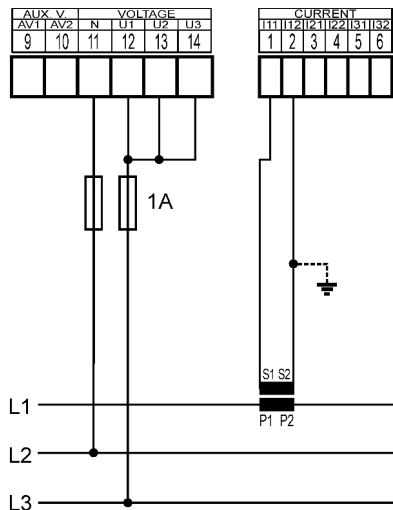
Síť IT typ zapojení 1D3
