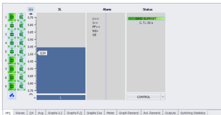
Indikace běžící podpory sítě v programu ENVIS/DAQ
