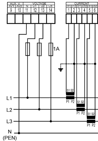
Síť TN
