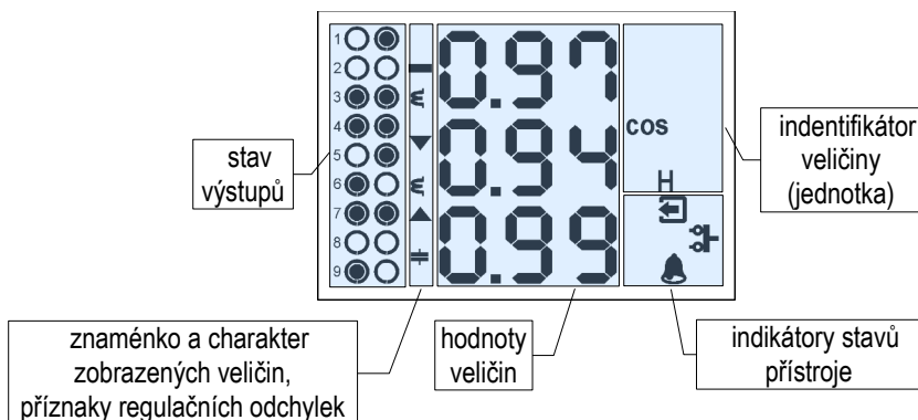
Obr. 4.1 : Příklad zobrazení okamžitých fázových účinnků
