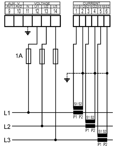
Síť IT
