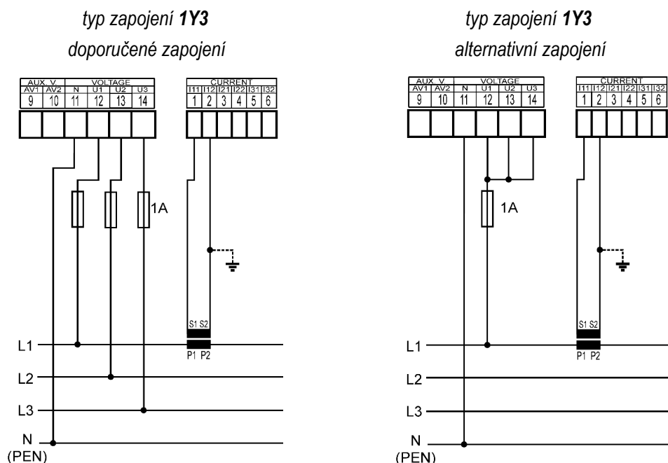
Obr. 4.22 : Jednofázové připojení k sítím se středním vodičem – příklady zapojení
